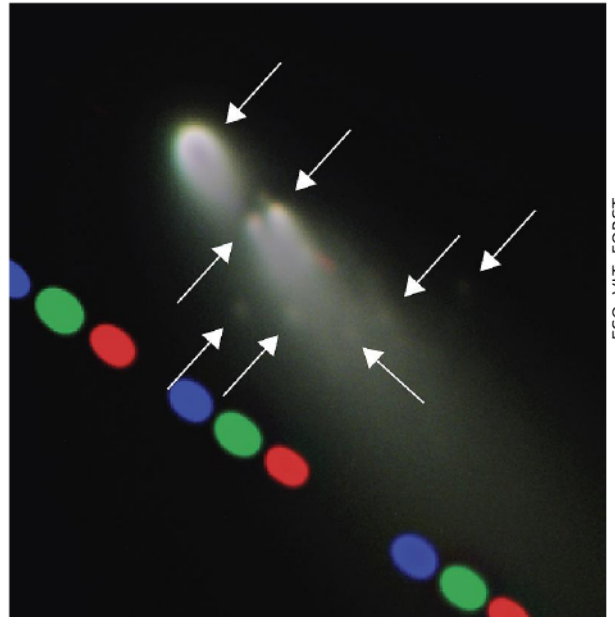
Fragmenty komety Schwassmann-Wachmann 3. Strzałki wskazują fragmenty różnej wielkości. Kropki na dole to obrazy pobliskich gwiazd sfotografowanych w różnych filtrach w czasie robienia zdjęcia.
