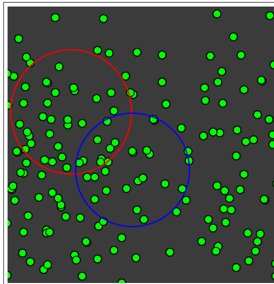
Rysunek 5: PROBLEM Z METODĄ ORBITY ŚREDNIEJ.
