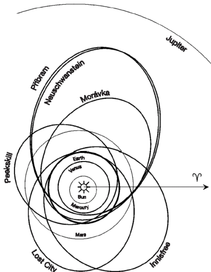
Orbita meteorytu Neuschwanstein w porównaniu z orbitą meteorytu Pribram
