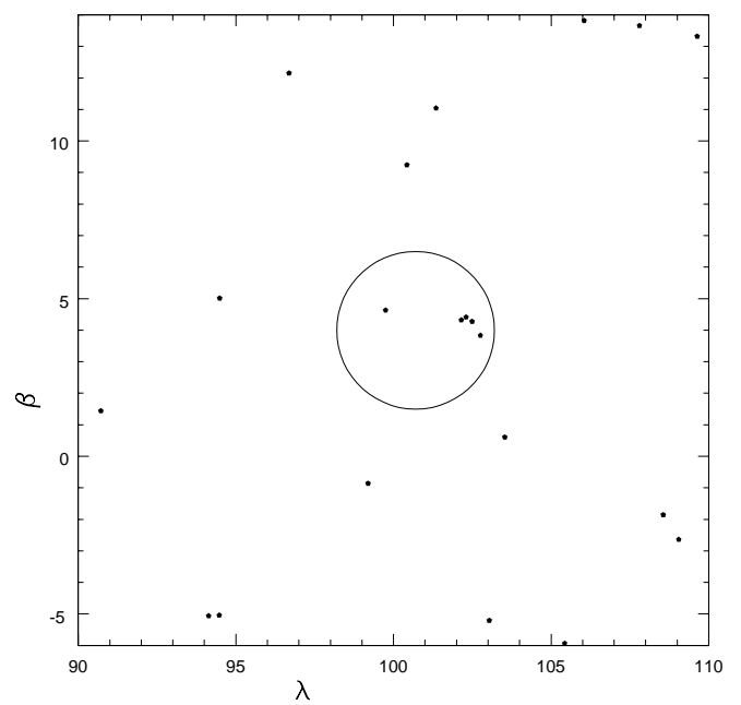
Rys.5. \epsilon -Geminidy
