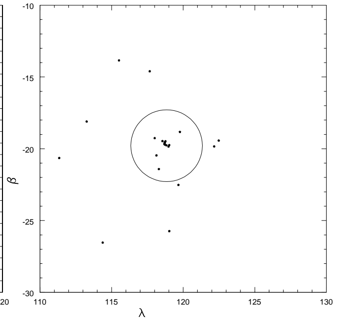
Rys.3. \alpha -Monocerotydy
